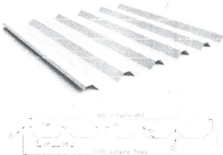
Figura 11 – imagem telha metálica trapezoidal TP40-980
