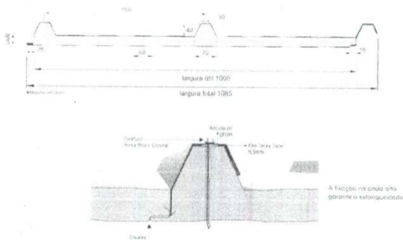
Figura 10 – imagem telha termoacústica
