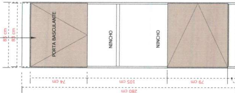
03 - VISTA 2 MB40 ESCALA.....1/20
