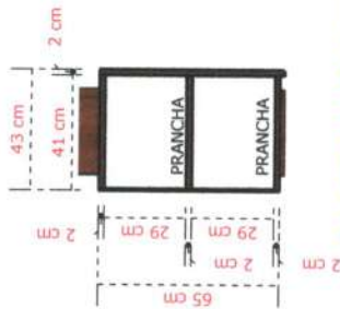
04 - CORTE LATERAL MB41 ESCALA.....1/20
