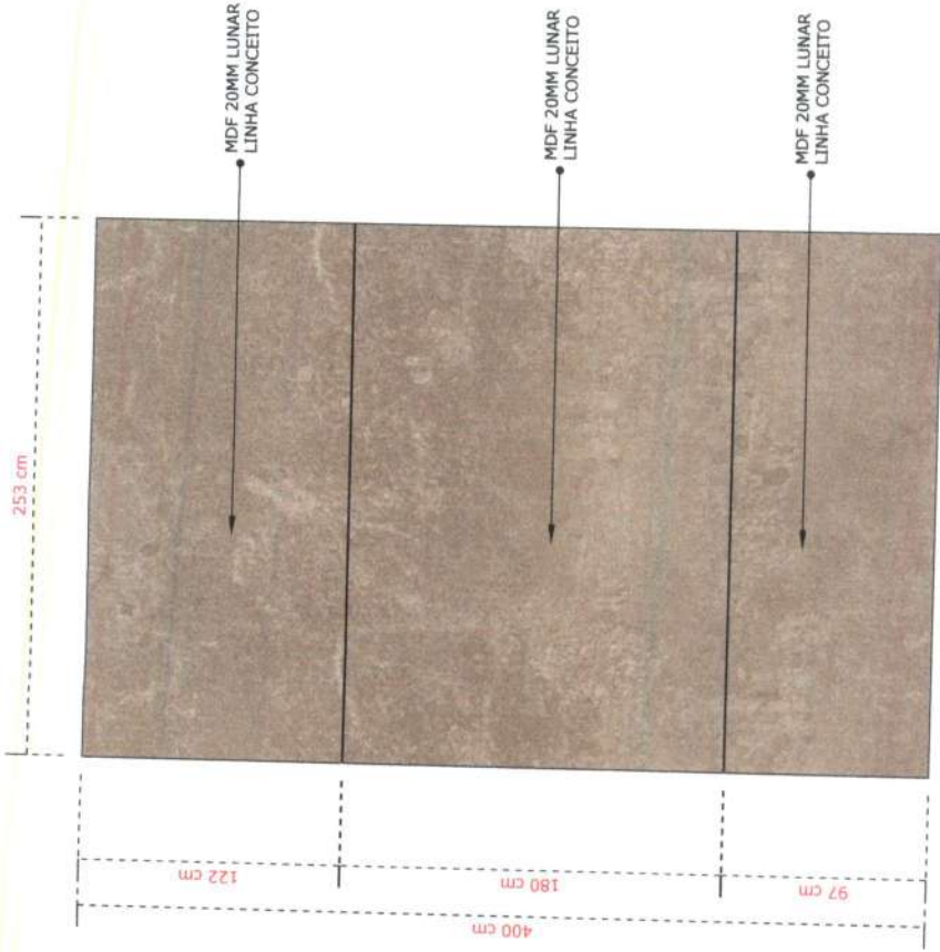
02- VISTA 1 MB31 ESCALA.....1/30
