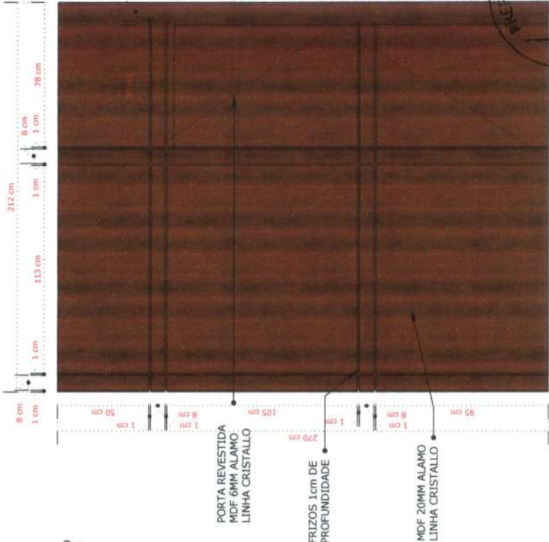
08- VISTA 2 MB19 ESCALA.....1/20
