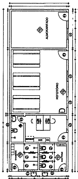
02 PLANTA BAIXA CANTEIRO DE OBRAS ESCALA 1/50
