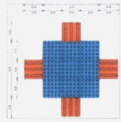
5 DET PISO PODOTÁTIL INTERNO 4 DIREÇÕES
