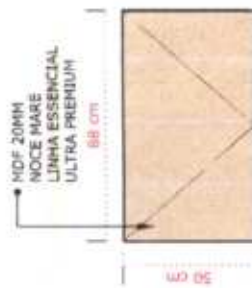
02- VISTA FRONTAL MB28 ESCALA.....1/20
