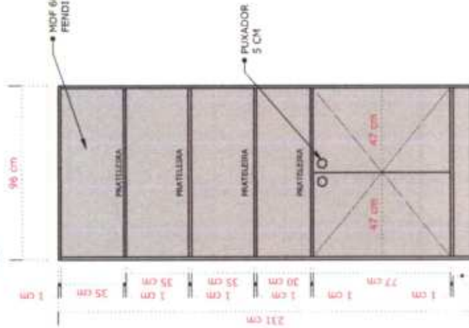
03 - VISTA FRONTAL MB9 ESCALA.....1/20
