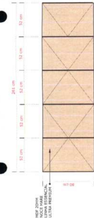
02- VISTA FRONTAL MB29 ESCALA.....1/20
