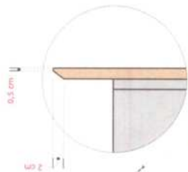
05- DET. 4 GAVETA MB25 ESCALA.....1/20
