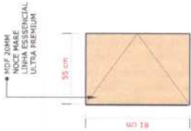
04- VISTA FRONTAL MB28 ESCALA.....1/20
