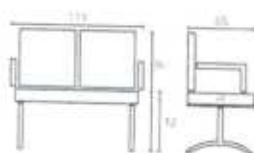
Medidas da longarina BLM 206:
