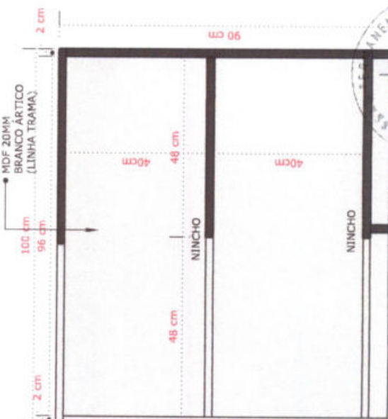
05 - CORTE LATERAL MB10 ESCALA.....1/10
