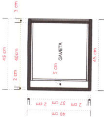
02 - PLANTA BAIXA MBS ESCALA.....1/10
