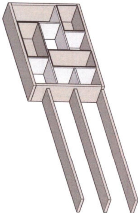
01 - ISOMÉTRICO MB7 ESCALA.....1/10
