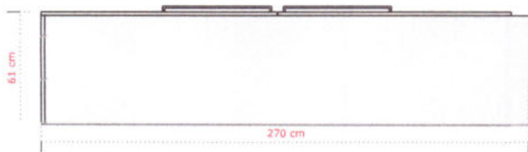
07 - VISTA LATERAL MB33 ESCALA.....1/20
