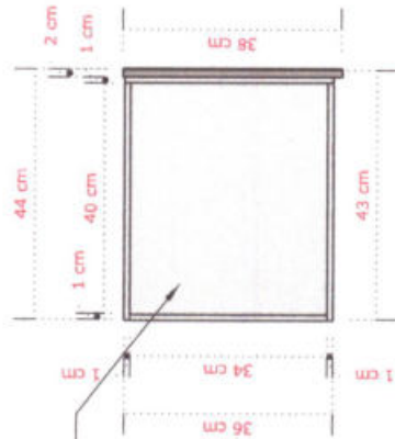
06 - DET. GAVETA MB3-VS ESCALA.....1/10
