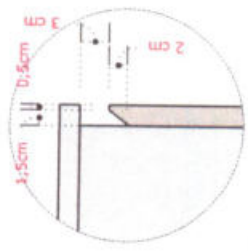
03 - DET. PUXADOR CAVA MB11 ESCALA.....1/10
