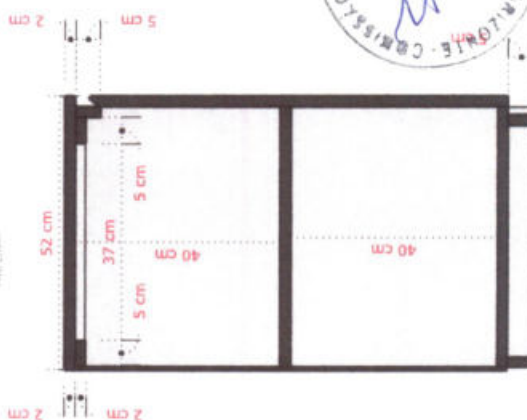
04- CORTE LATERAL MB11 ESCALA.....1/10
