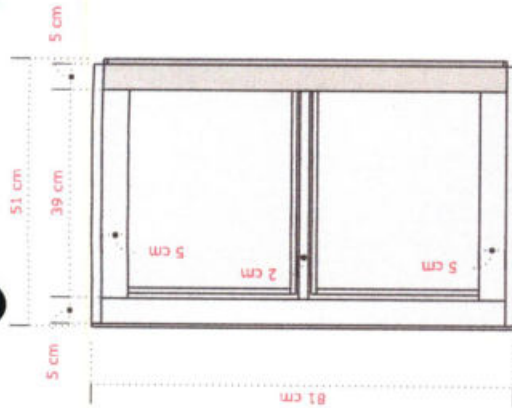
02 - VISTA SUPERIOR MB3 ESCALA.....1/10
