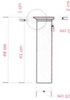
07 - DET. GAVETA MB3-VL ESCALA.....1/10
