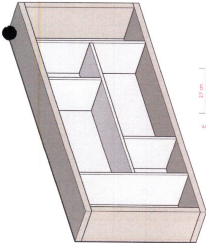
01 - ISOMÉTRICA MB9 ESCALA.....1/10
