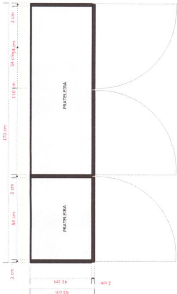
02 - PLANTA BAIXA MB18 ESCALA.....1/10
