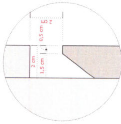
02 - DET. PUXADOR CAVA MB27 ESCALA.....1/1
