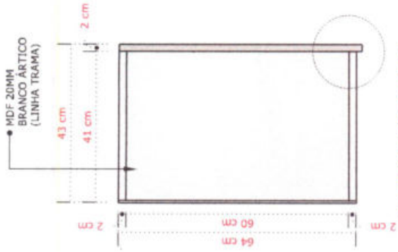
02 - VISTA LATERAL MB18 ESCALA.....1/10
