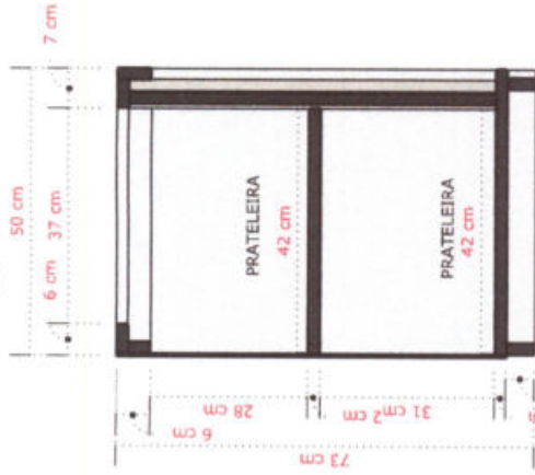
03 - CORTE LATERAL MB1 ESCALA.....1/10
