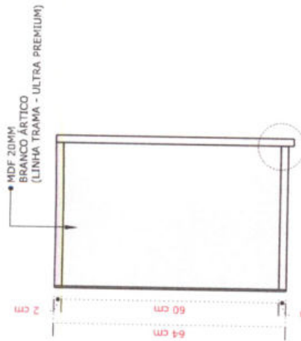
01 - VISTA LATERAL MB21 ESCALA.....1/10
