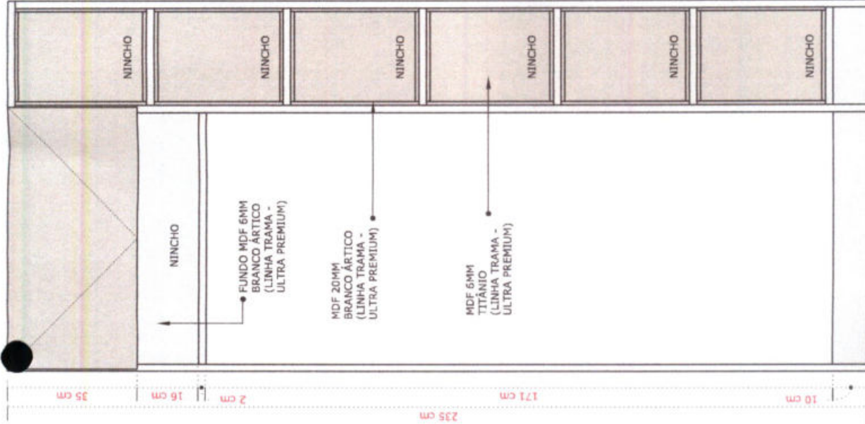
02 - VISTA FRONTAL MB29 ESCALA.....1/10
