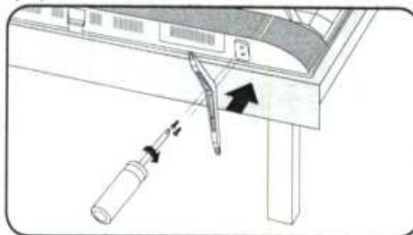
Forma CORRETA de instalação.
