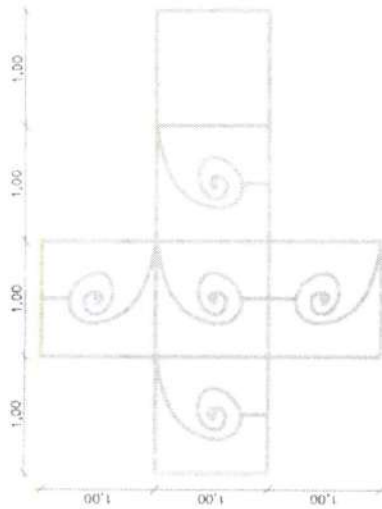
03- DETALHE PRESENTE O ESCALA 1/10
