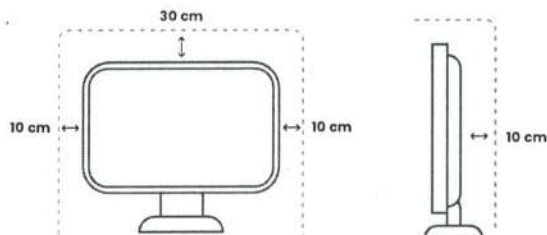
INSTALAÇÃO COM BASE
