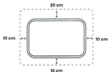
INSTALAÇÃO NA PAREDE
