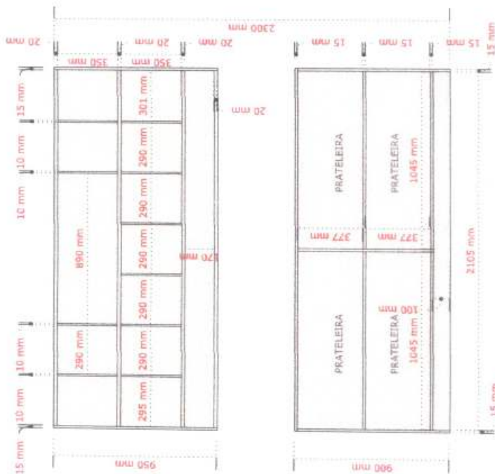
03 - VISTA INTERNA (ARMÁRIO M06)
