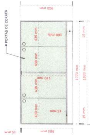
03 - VISTA FRONTAL (BANCADA M02)
