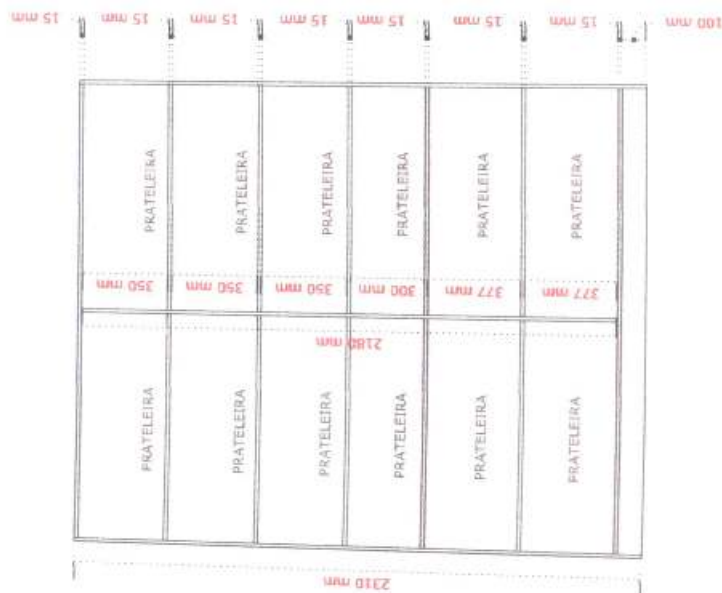
03 - VISTA INTERNA (ARMÁRIO M10)
