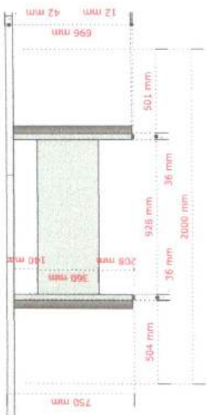
02 - VISTA FRONTAL (MESA M04)
