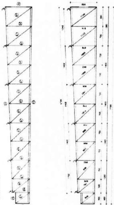
DETALHE VM1 Escala 1/20 (FABRICAÇÃO EM FERRÃO)
