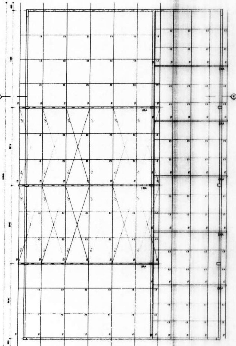
PLANO DE TERÇAS
