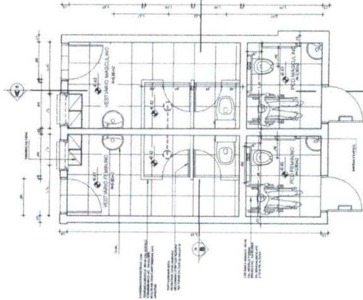
04 PLANTA BARRA - VESTIÁRIO
