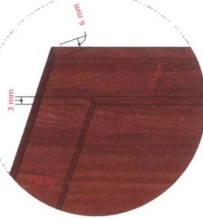
04 - DET. 01 ESCALA.....1/1
