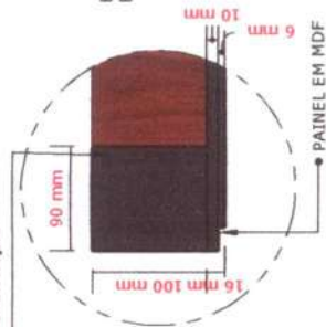
03 - DETALHE 1 ESCALA.....1/5
