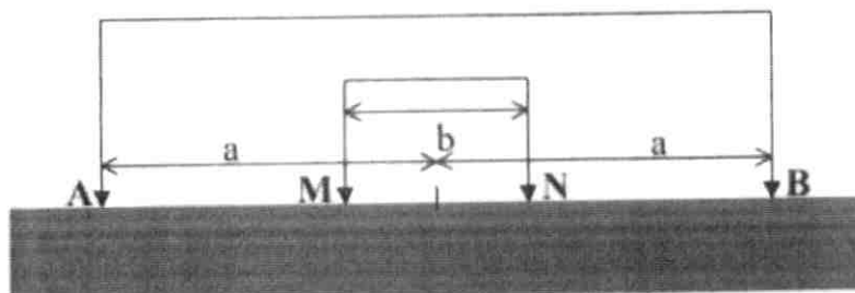
Figura 8 – Disposição dos eletrodos de corrente A e B e dos eletrodos de medida da diferença de potencial para o arranjo Schlumberger.
