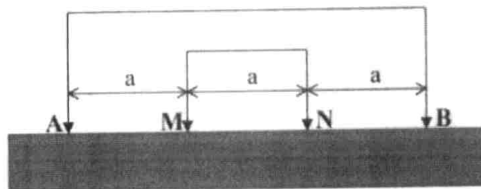
Figura 7 – Disposição dos eletrodos de corrente A e B e dos eletrodos de medida da diferença de potencial para o arranjo Wenner.
