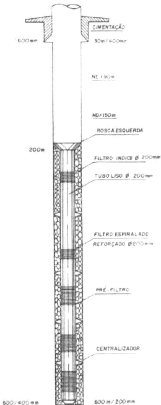
PERFIL CONSTRUTIVO
