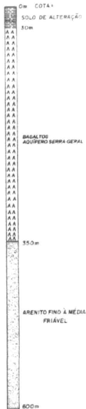
PERFIL GEOLOGICO
